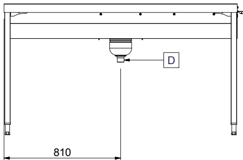
Zij aanzicht
